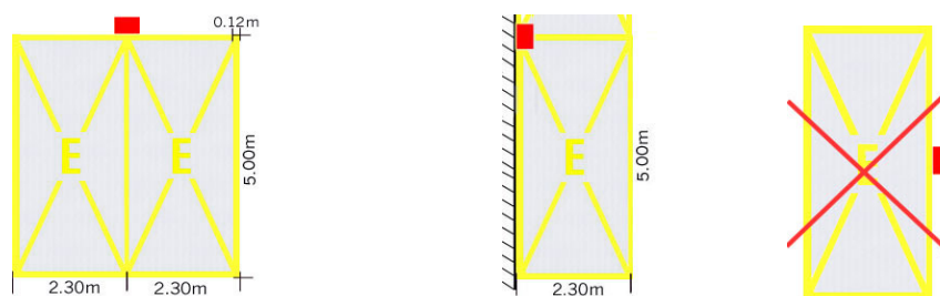
Abbildung 2: Stellfläche/Parkfeld EV, PHEV
