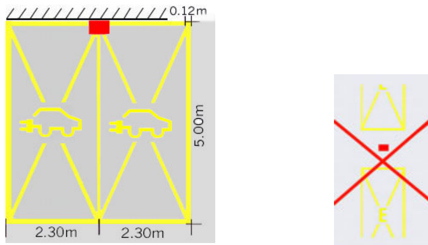
Abbildung 2: Stellfläche/Parkfeld EV, PHEV
